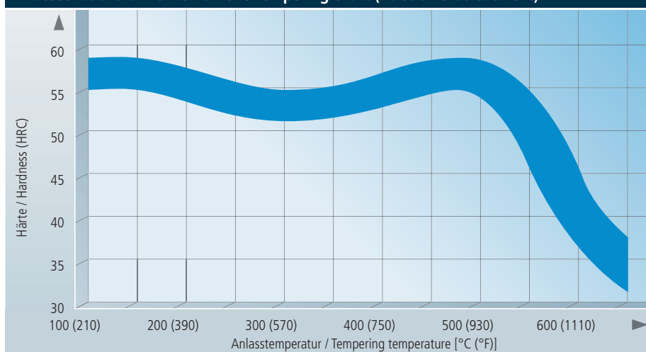
Anlassschaubild ohne Tiefkühlen / Tempering chart (no sub-zero treatment)
