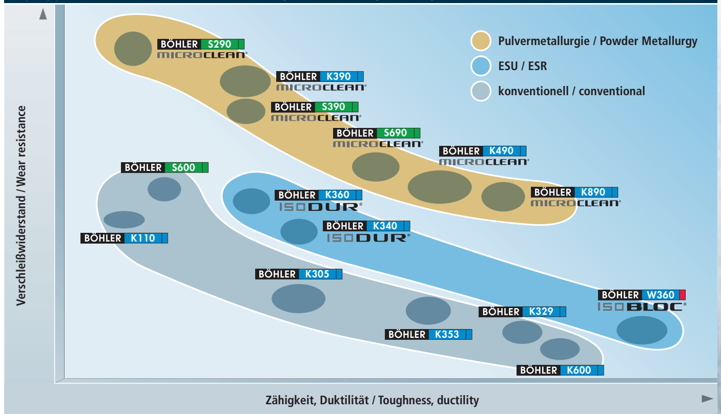
Eigenschaftsprofil von BÖHLER Kaltarbeitsstählen in Abhängigkeit der Herstelltechnologien / Property profile of BÖHLER cold work steels according to manufacturing technologies
